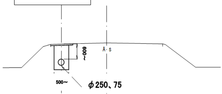
標準管路横断面図
