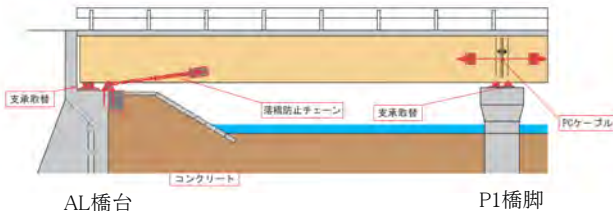
AL橋台
